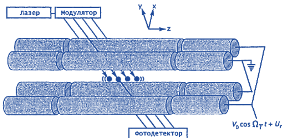
Рис. 3.5. Схема квантового компьютера, реализованного с помощью ионных ловушек
