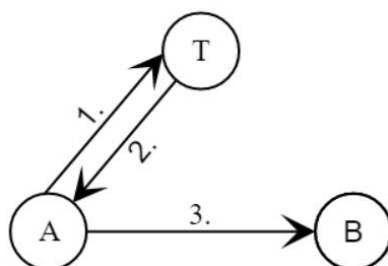
Рис. 5.22. Формирование нового сессионного ключа
