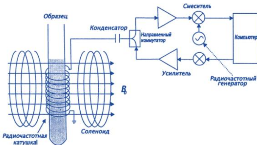
Рис. 3.13. Схематическая диаграмма ЯМР-спектрометра
