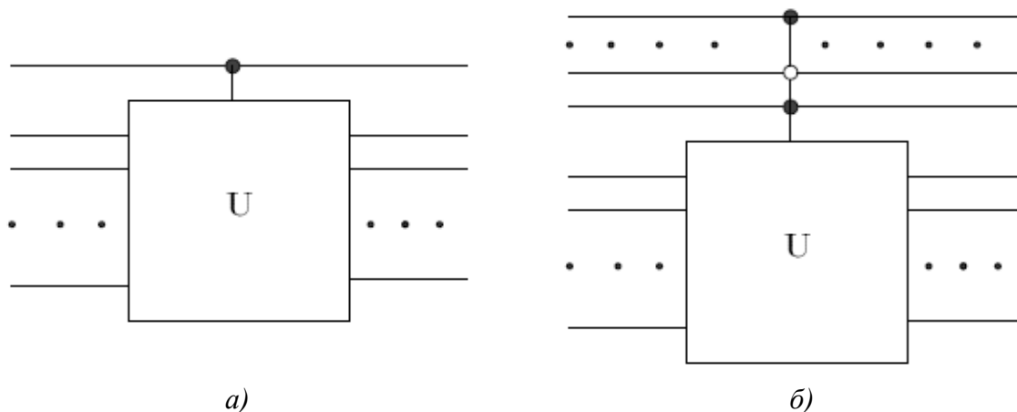
Рис. 1.7. Унитарный гейт:
