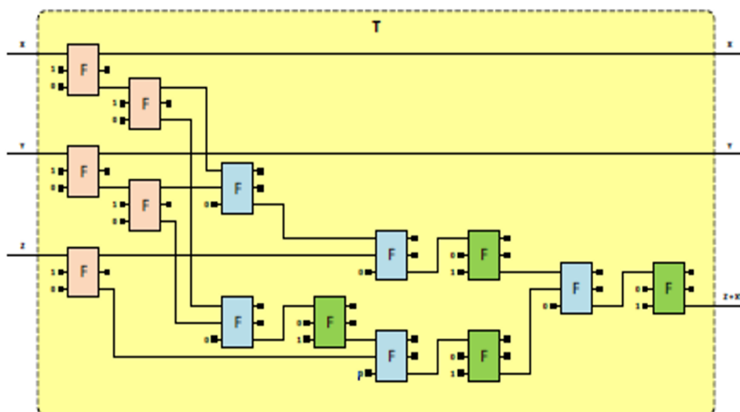
Рис. 1.9. Диаграмма, демонстрирующая один из вариантов выражения элемента Тоффоли через элемент Фредкина (красным цветом показаны элементы FAN OUT , синим – И , зелёным – НЕ )
