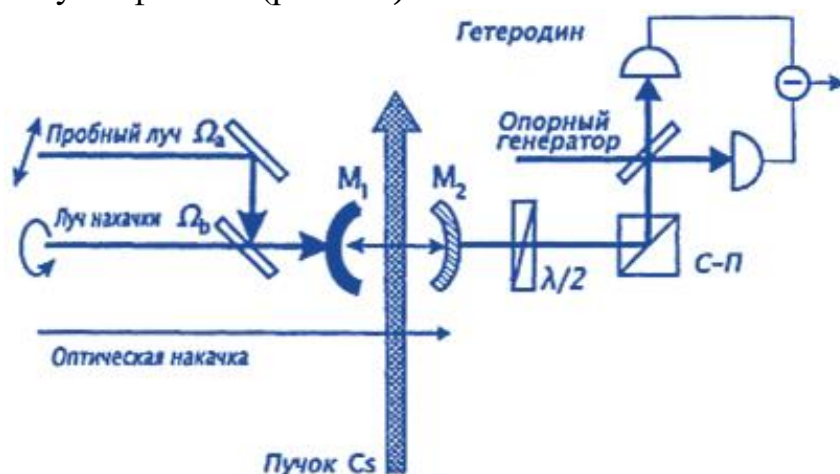
Рис. 3.4. Схема экспериментальной установки для реализации элементарного квантового логического элемента
