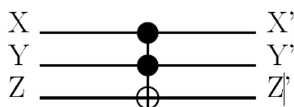
Рис. 1.8. Гейт Тоффоли для случая квантового параллелизма
