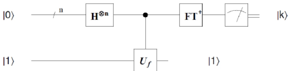
Рис. 2.6. Квантовая схема для измерения фазы оператора R_z[\varphi]
