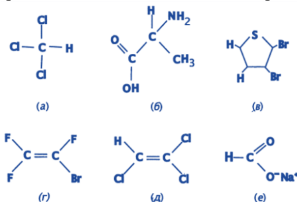
Рис. 3.17. Примеры простейших молекул, использованных в экспериментах по реализации квантовых вычислений методом ядерного магнитного резонанса
