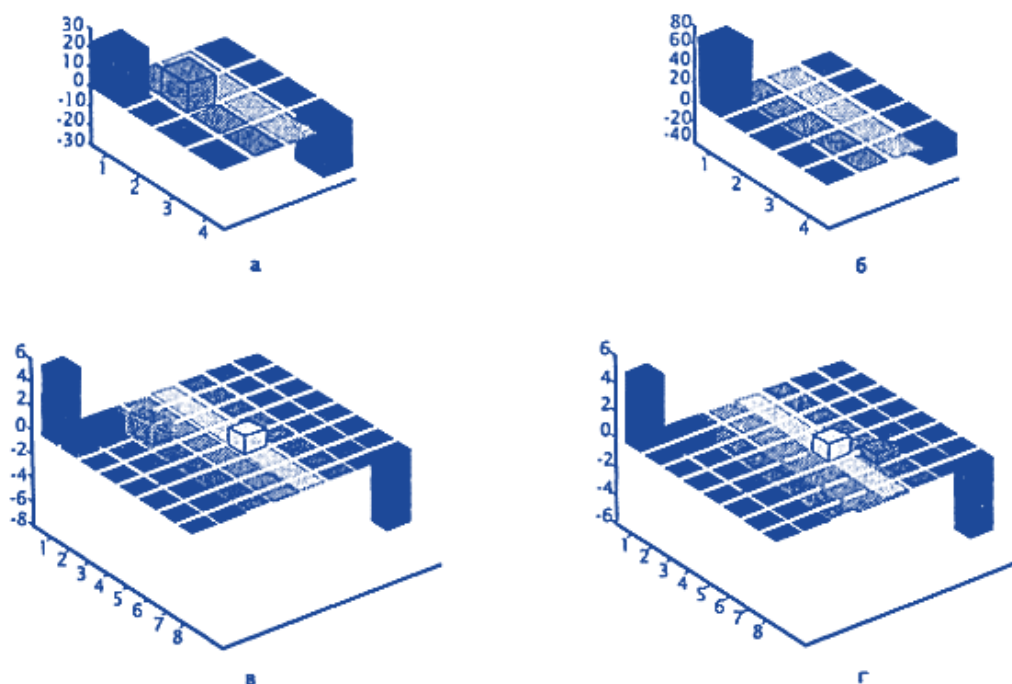
Рис. 3.14. Экспериментальное измерение матрицы плотности в разностной форме
