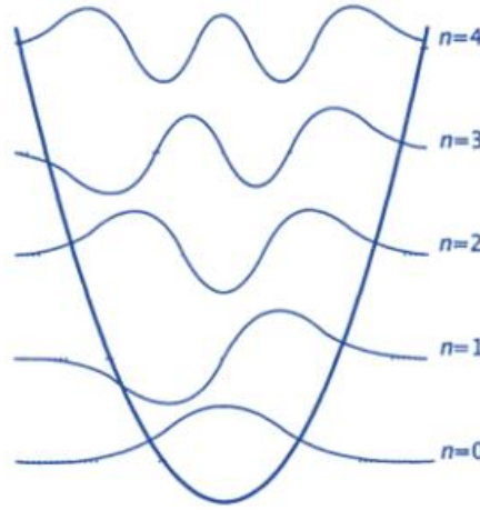
Рис. 3.1. Решения уравнения Шрёдингера
