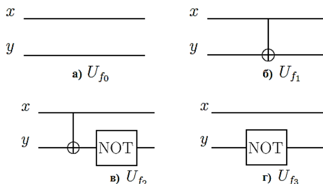
Рис. 2.1. Квантовое преобразование четырёх функций
