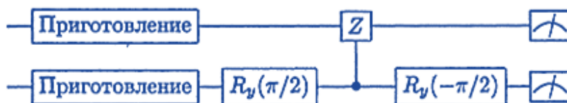
Рис. 3.11. Квантовая схема экспериментальной реализации операции C_{NOT} .
