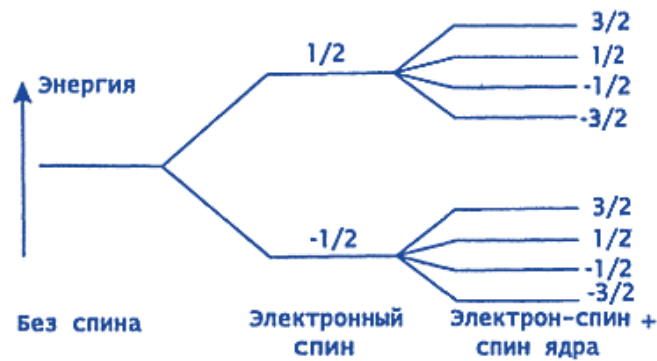
Рис. 3.6. Расщепление атомных уровней в магнитном поле
