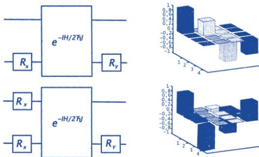
Рис. 3.15. Квантовые схемы, реализованные методом ЯМР
