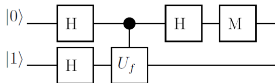
Рис. 2.2. Квантовая схема алгоритма Дойча
