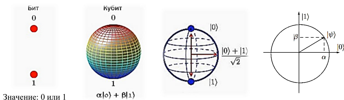
Рис. 1.1. Состояние кубита: единичный вектор в двумерном комплексном пространстве с базисом \{|0\rangle, |1\rangle\}
