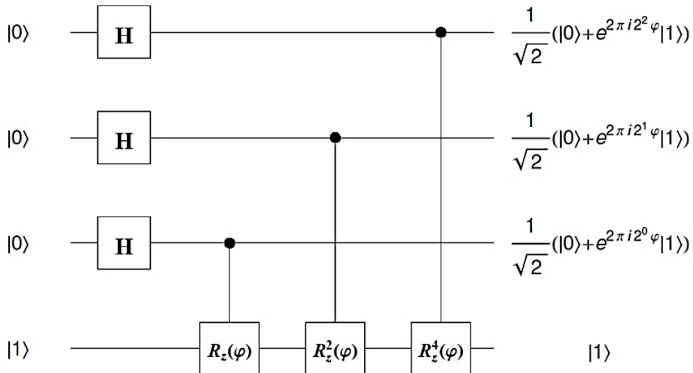
Рис. 2.5. Квантовая схема, приводящая квантовый регистр памяти
