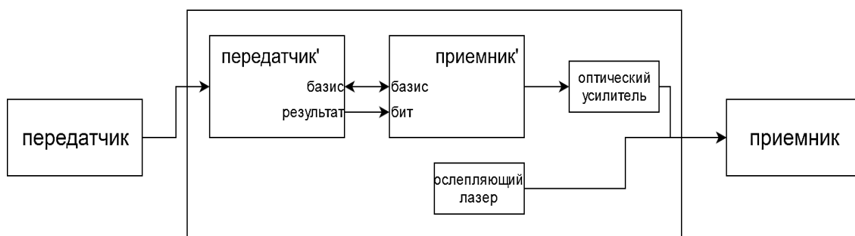
Рис. 5.2. Схема применения атаки с ослеплением детектора
