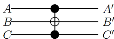
Рис. 1.6. Графическое изображение универсального квантового гейта Тоффоли
