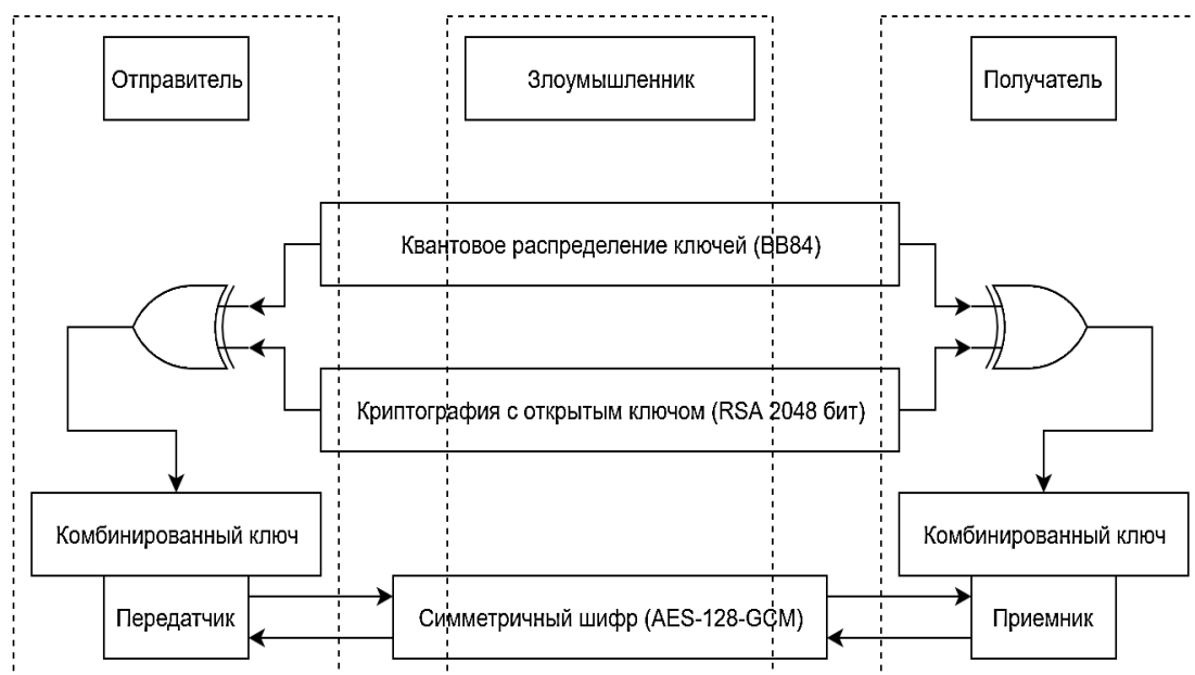
Рис. 5.1. Схема передачи данных с квантовым распределением ключей
