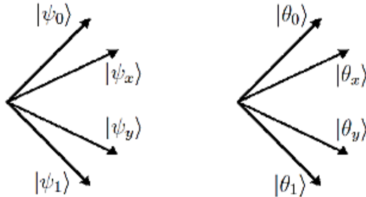
Рис. 4.1. Симметричное расположение базисных векторов |\psi_0\rangle , |\psi_1\rangle , |\theta_0\rangle , |\theta_1\rangle относительно квантовых состояний в пространстве перехватчика Евы
