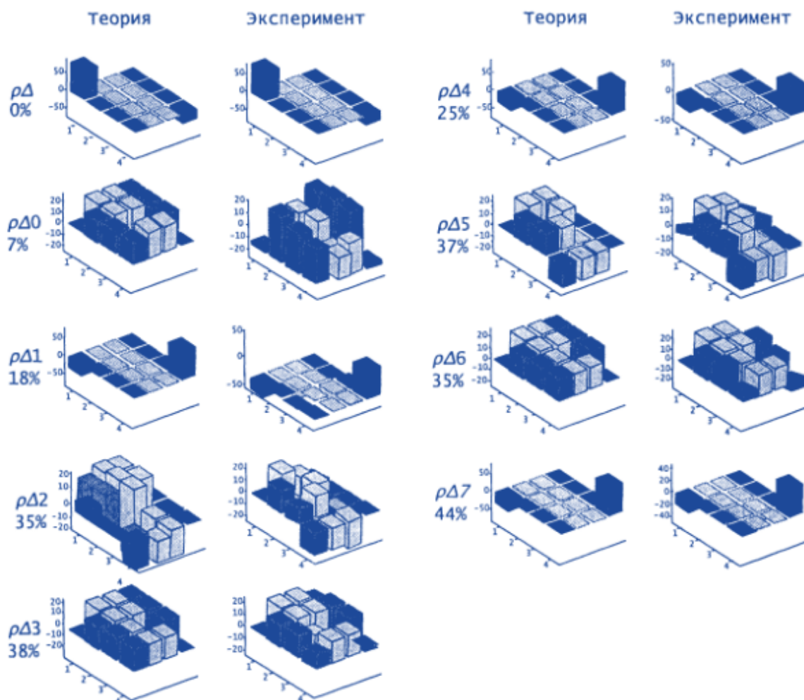
Рис. 3.16. Матрицы плотности в разностной форме для семи итераций алгоритма Гровера, полученные теоретически и экспериментально на спинах водорода и углерода в хлороформе
