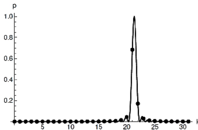
Рис. 2.7. Вероятности получения различных результатов измерения фазы в случае регистра из 5 кубитов
