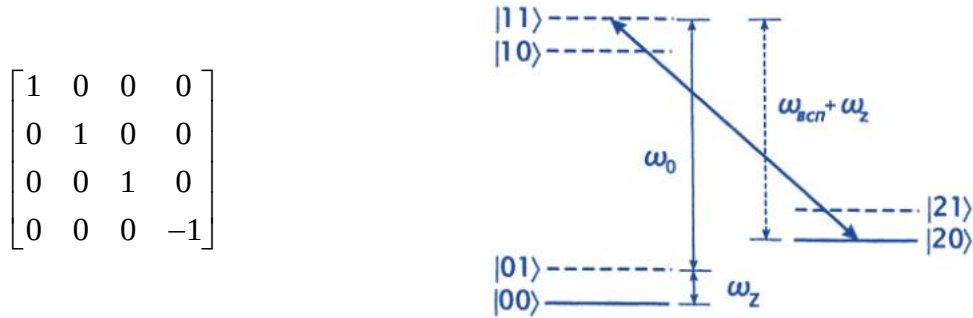
Рис. 3.9. Уровни энергии трёхуровневого атома, помещенного в ионную ловушку
