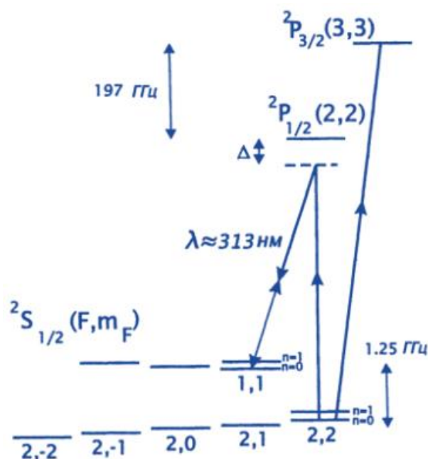
Рис. 3.10. Уровни энергии иона {}^9\text{Be}^+ в ионной ловушке
