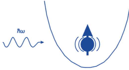
Рис. 3.7. Модель иона в ловушке: одиночная двухуровневая частица в параболическом потенциале, взаимодействующая с электромагнитным полем
