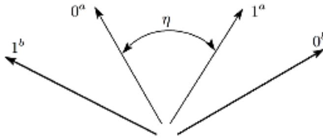
Рис. 4.2. Геометрия квантовых состояний в протоколе SARG04. Состояния 0 и 1 из разных базисов взаимно ортогональны
