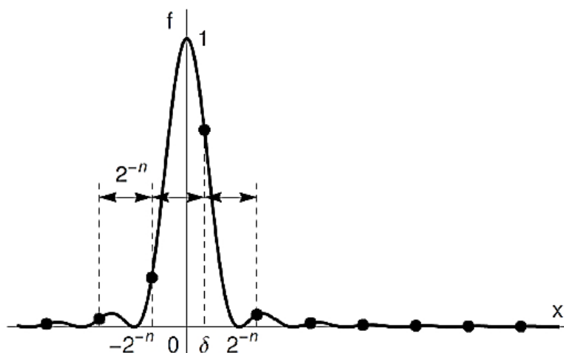
Рис. 2.4. График функции y = f(x) и значения функции в точках x = \varphi - \frac{j}{2^n}
