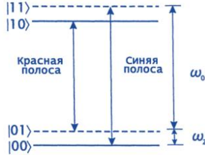
Рис. 3.8. Схема уровней энергии для модели ионов в ловушке, демонстрирующая красные и синие боковые полосы, возникающие за счёт испускания или поглощения одного фонона
