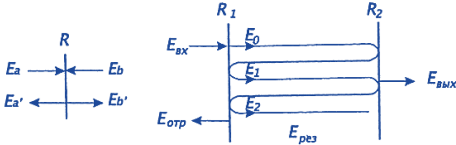
Рис. 3.3. Схема работы резонатора Фабри – Перо
