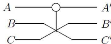
Рис. 1.5. Универсальный квантовый гейт Фредкина
